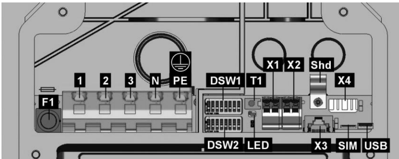
Abbildung 2: Anschlussübersicht KEBA-Ladestationen
