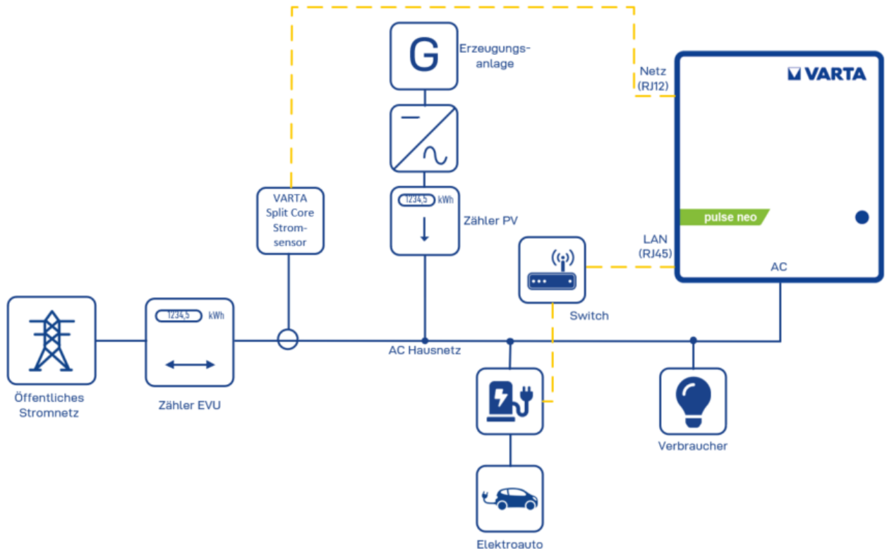
Abbildung 1: Systemübersicht VARTA pulse neo Ladestationsinteraktion
